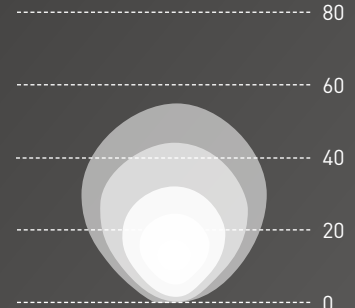
INTELLiLight® / 2900 lm Breit Symmetrisch (Nahfeld)
