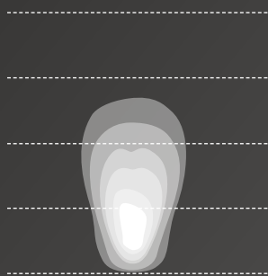
INTELLiLight® / 2900 lm Asymmetrisch (Nahfeld)
